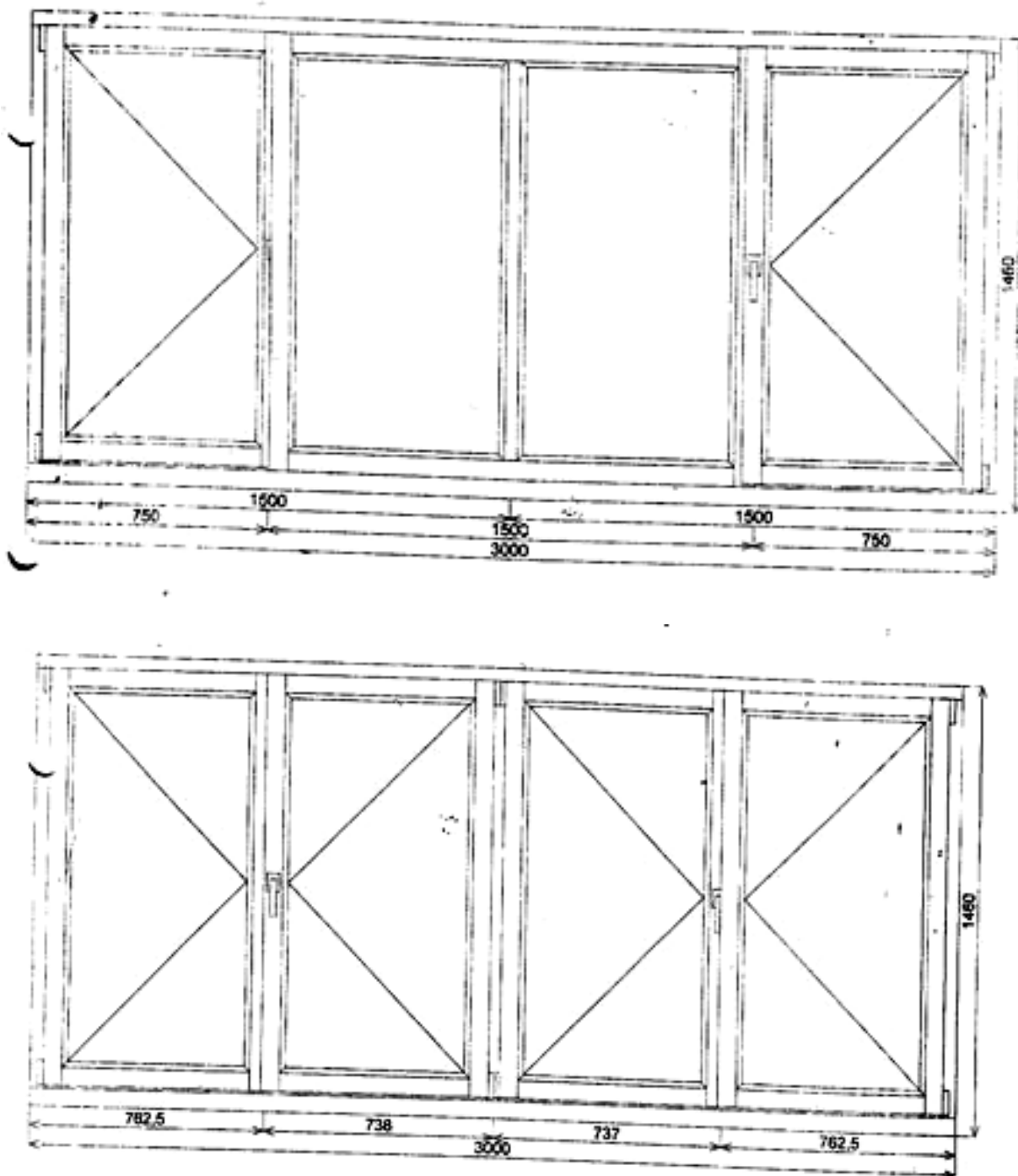
Рисунок 3 – Эскизы конструкций заполнения оконных проёмов
