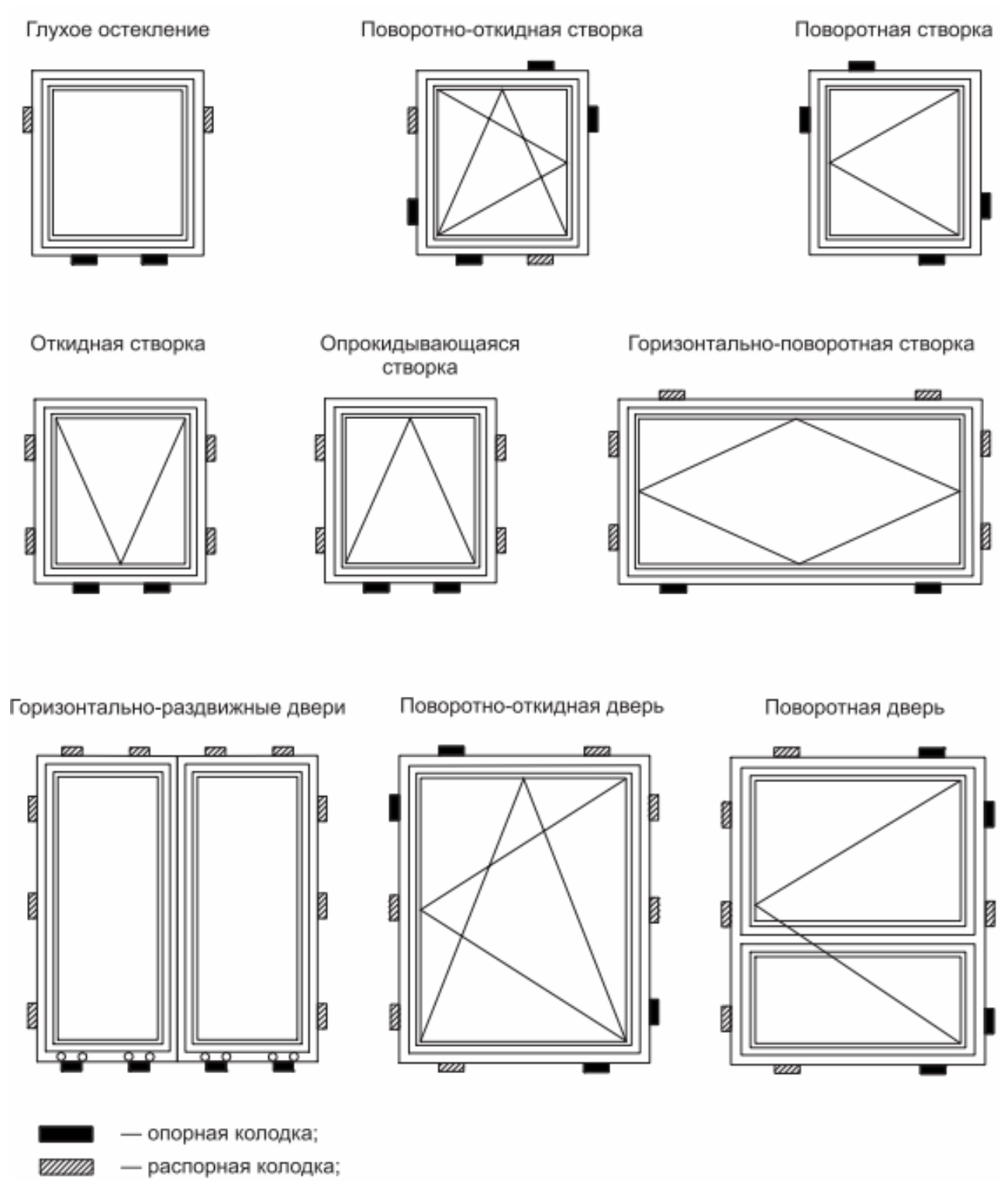
Рисунок 2 – Примеры расположения колодок и креплений
